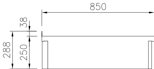
Zij aanzicht
